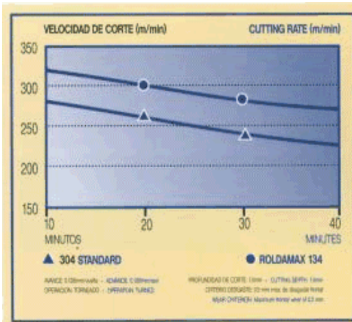
VIDA DE LA CUCHILLA EN FUNCIÓN DE LA VELOCIDAD DE CORTE
