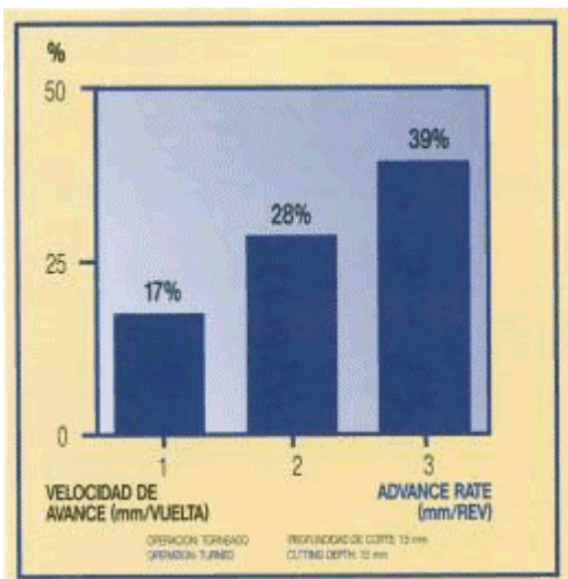
INCREMENTO EN LA VELOCIDAD DE CORTE DEL ROLDAMAX SOBRE EL 304 ESTANDAR EN FUNCIÓN DE LA VELOCIDAD DE AVANCE
