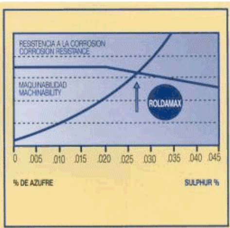
MAQUINABILIDAD Y RESISTENCIA A LA CORROSION EN FUNCIÓN DEL CONTENIDO EN AZUFRE
